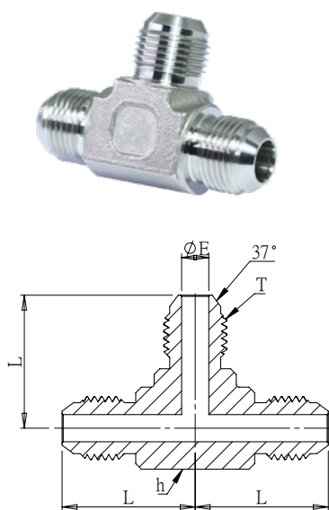
油壓 37°三通由任接頭 Union Tee
